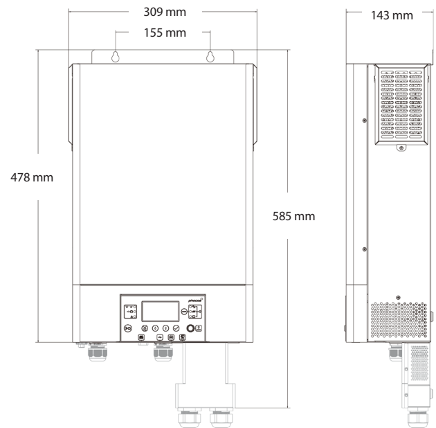
PSW-H-5KW-120/48V, PSW-H-6.5KW-120/48V and PSW-H-8KW-230/48V*
