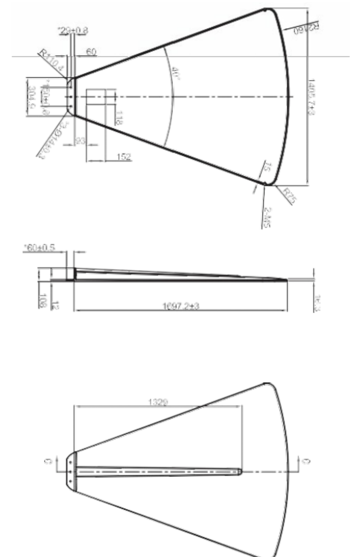
Abbildung 2. Abmessung PV Blatt
